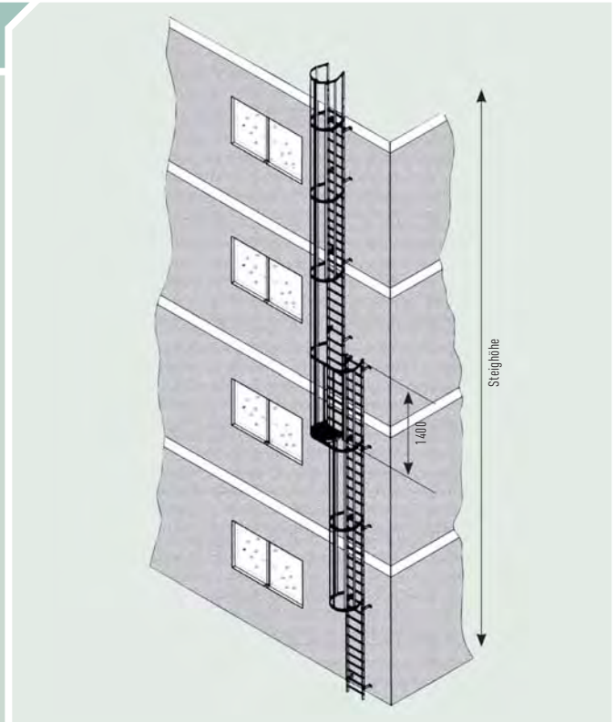
Rückenschutzbügel für versetzte Ausführung.
