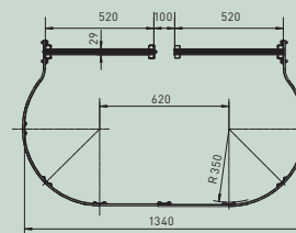
Rückenschutzbügel für versetzte Ausführung.
